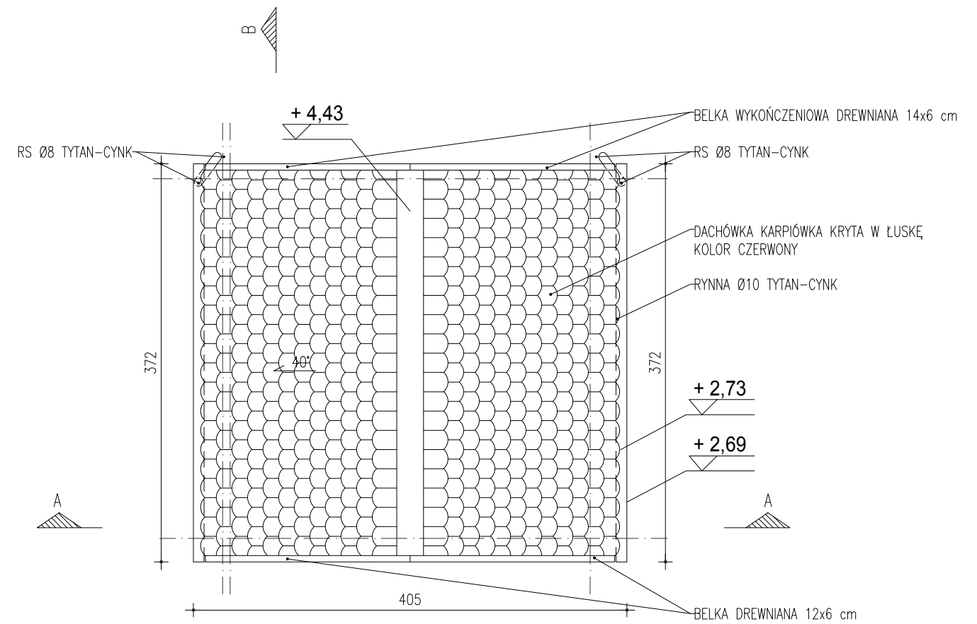
RZUT DACHU
