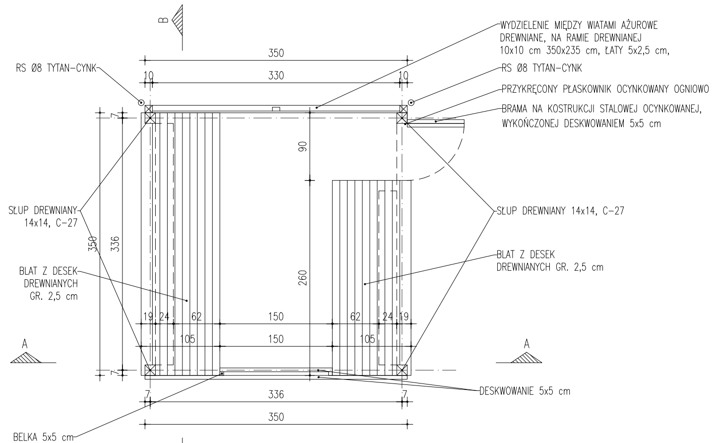
RZUT
