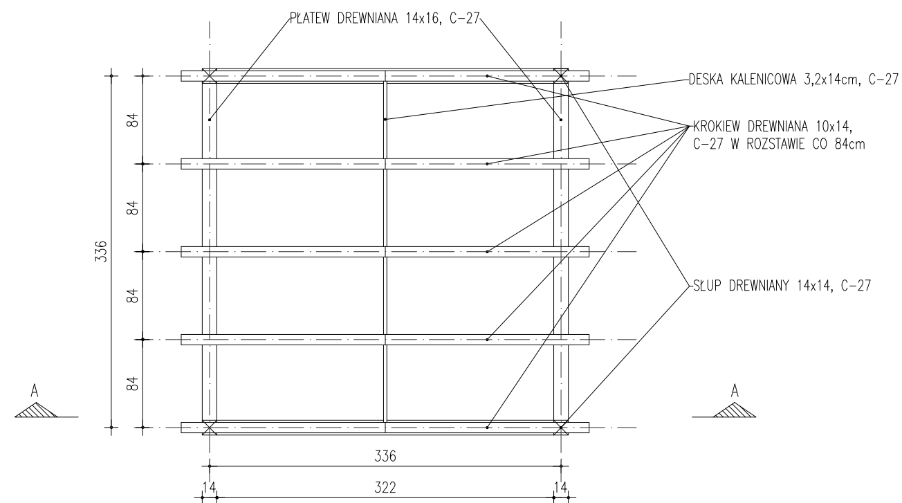
RZUT WIĘŻBY DACHOWEJ
